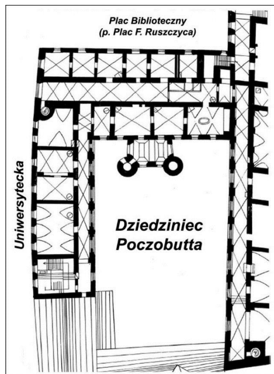
Zachodnie i północne skrzydło Dziedzińca Poczobutta. Plan II piętra.
