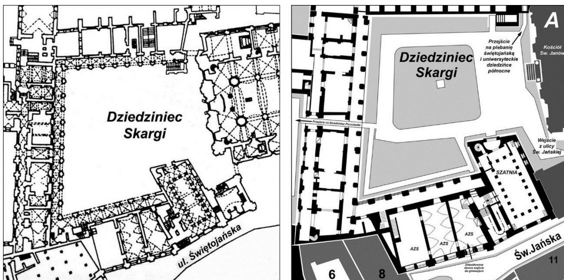
Dziedziniec Skargi (Wielki). Po lewej rzut parteru z 1997 r. (Źródło: opracowanie E. Małachowicza na podstawie KPDA). Po prawej skrzydło południowe i zachodnie — plan pomieszczeń parteru z przyziemiem. (Opracowanie własne autora).
