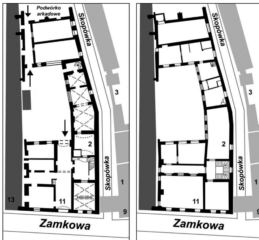
Zespół domu przy ulicy Zamkowej 11/róg Skopówki (rzut parteru i I piętra). (Opracowanie własne autora na podstawie planów ze zbiorów archiwum w Wilnie m.in.: VAA, F. 1019, ap. 11, b. 6635, VAA, F. 2, B. 118-22).
