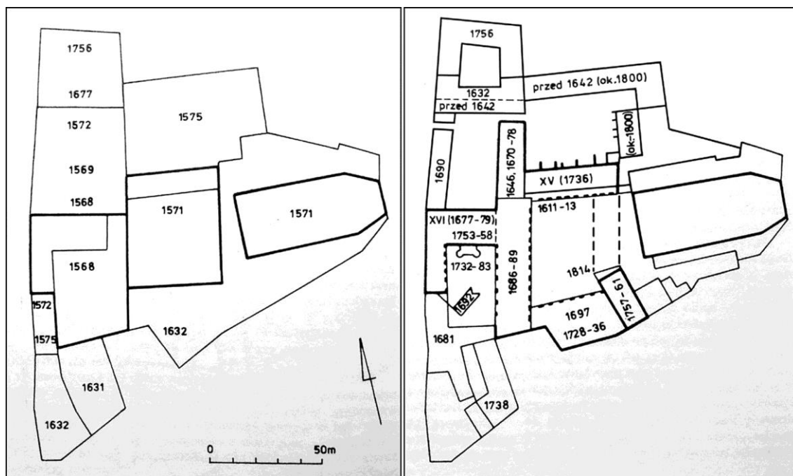
Kompleks główny uniwersytetu w Wilnie z datami przyłączania poszczególnych zespołów budynków oraz ich przebudowy w następnych latach. Ostatnią z dat jest 1814 rok, kiedy przebudowano elewację Auli. (Źródło: E. Małachowicz, Wilno. Dzieje... , s. 149-150).
